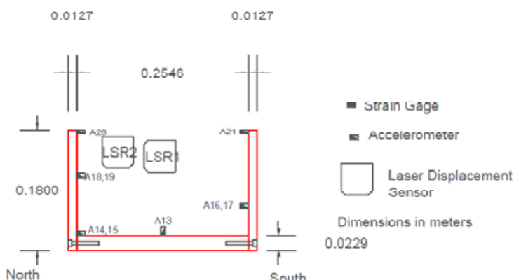
Σχήμα 4: Τομή τοίχου αντιστήριξης και διάταξη μετρητικού εξοπλισμού.
