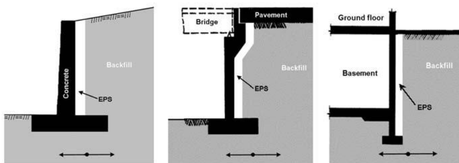
Σχήμα 1: Μόνωση έναντι οριζόντιας σεισμικής ώθησης, σε κατασκευές εδαφικής αντιστήριξης με συμπιεστό παρέμβλημα γεωαφρού EPS.
