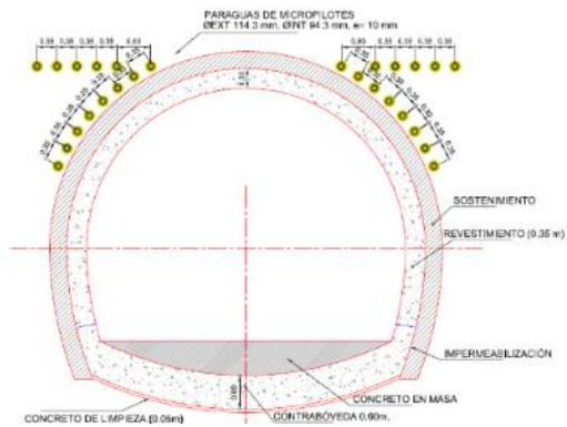
Figura 11. Diseño de sostenimiento tipo 2 en la galería técnica tipo GE-II, en zona de brechas, referencia 3
