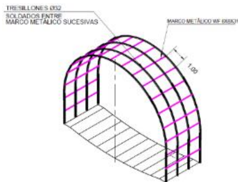
Figura 12. Diseño de marcos metálicos para las galerías de evacuación y técnicas tipo GE-II y GT-II, en zona de brechas, referencia 3.
