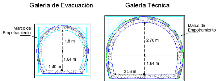
Figura 6. Diseño para las galerías de evacuación y técnica tipo GE-I y GT-I, en la etapa previa al corte de las dovelas, referencia 3.
