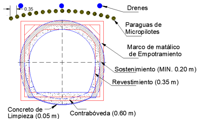
Figura 10. Diseño para las galerías de evacuación tipo GE-II en zona de brechas, referencia 3.
