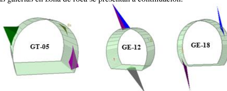
Figura 13. Análisis de cuñas para las galerías GT-05, GE-12 y GT-18, referencia 5.
