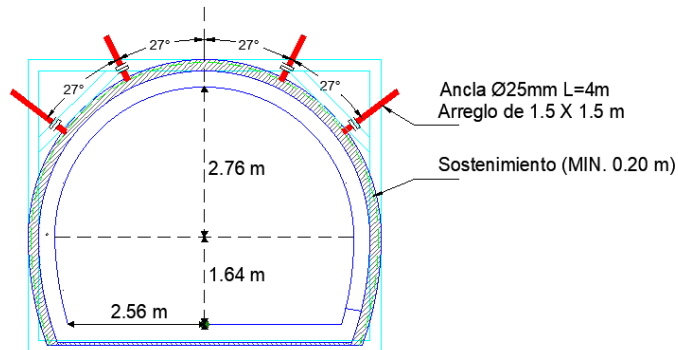
Figura 7. Diseño de arreglo de anclas y concreto lanzado para las galerías de evacuación y técnicas tipo GE-I y GT-I, referencia 3 y 5.
