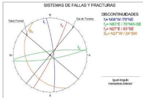
Figura 5. Estereograma con las orientaciones de los sistemas principales de fallas y fracturas del bitúnel, referencia 2.
