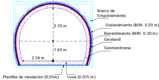
Figura 9. Tratamiento de impermeabilización con geotextil y geomenbrana, referencia 3.
