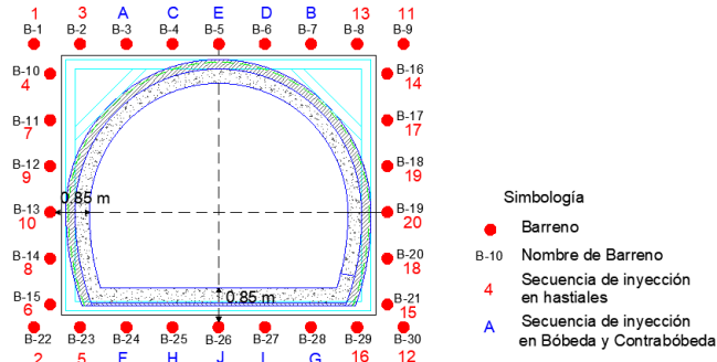
Figura 8. Diseño de plantilla de barrenos de inyección para tratamiento de impermeabilización previo al corte de las dovelas, referencia 2 y 3.
