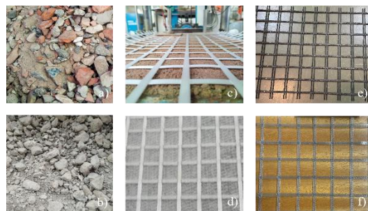
Figure 10: Materials used: a) RMA; b) RCA; c) GGRBv; d) GCR; e) GGRUr; f) GGRBr.
